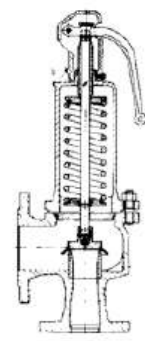
GSV...901 oA Kołpak zamknięty Dźwignia otwarta
