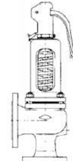
GSV...902 Kołpak otwarty Dźwignia otwarta
