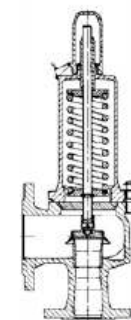
GSV...901 G Kołpak zamknięty Kaptur gazoszczelny
