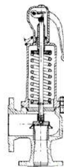
GSV...901 Kołpak zamknięty Dźwignia uszczelniona
