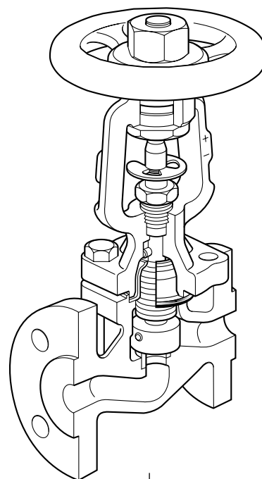
Przekrój BSA
